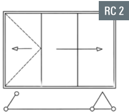
Typ 2 LS/1 RS.i
