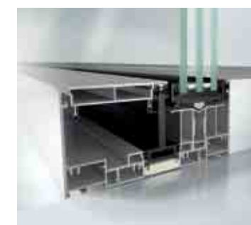
Schüco ASS 77 PD.HI Mechatronic/Manual
