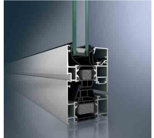
Schüco AWS 70.HI Schüco AWS 70.HI
