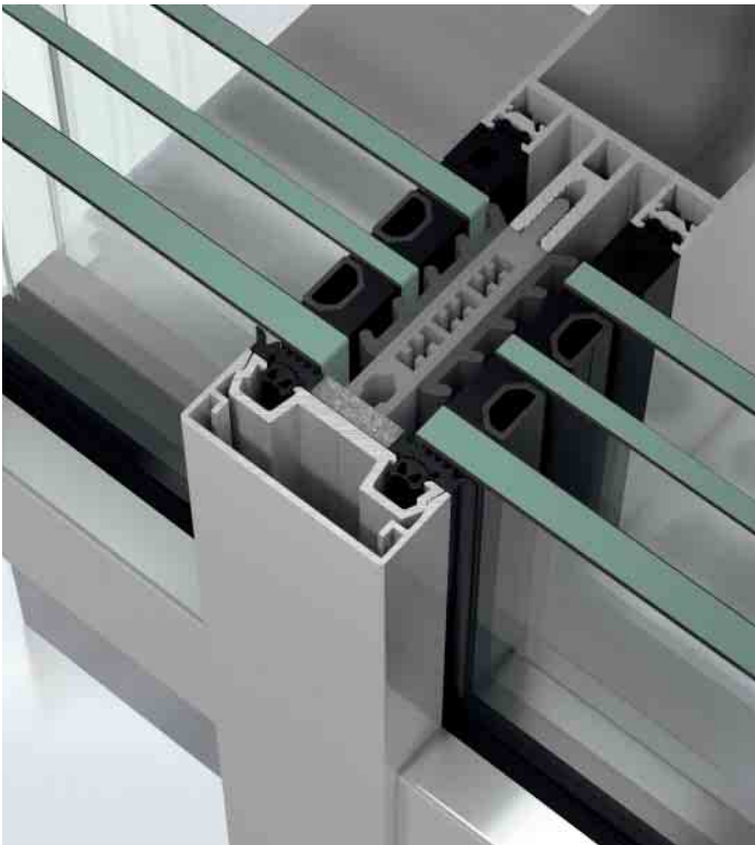
Schüco Fassade FWS 50.SI mit neuer passivhauszertifizierter Isolortechologie Schüco Façade FWS 50.SI with new passive house certified isolator technology
